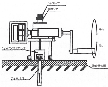
図1 アンカーピンの引抜き試験
